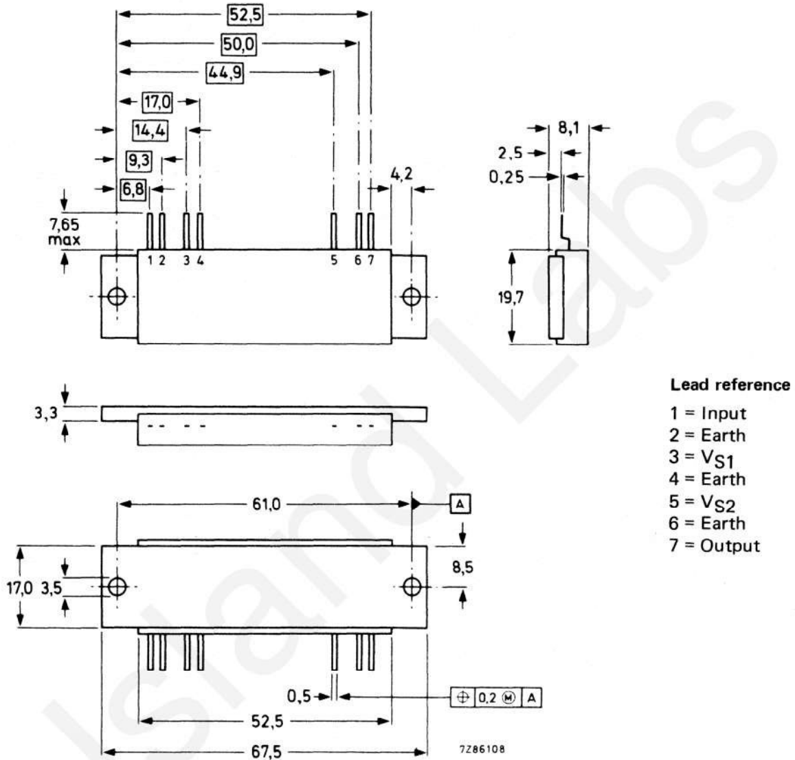
Fig. 15 SOT-132C.
